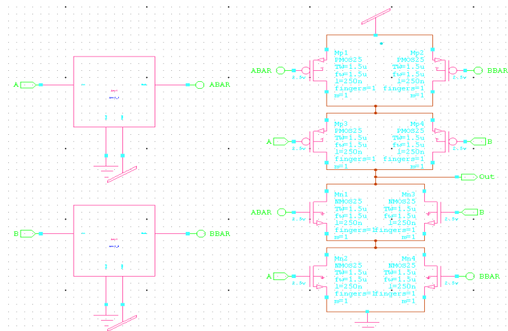
Fig3.3:XORSCHMATIC
